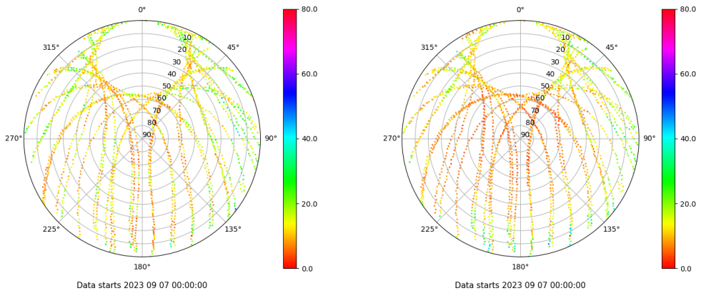
Skyplot for station ALOR. Parameter M1C Data file ALOR00ESP_R_2023250.xtr Skyplot for station ALOR. Parameter M2P Data file ALOR00ESP_R_2023250.xtr
