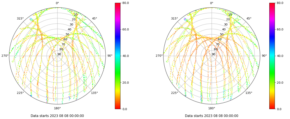
Skyplot for station ALOR. Parameter M1C Data file ALOR00ESP_R_2023220.xtr Skyplot for station ALOR. Parameter M2P Data file ALOR00ESP_R_2023220.xtr
