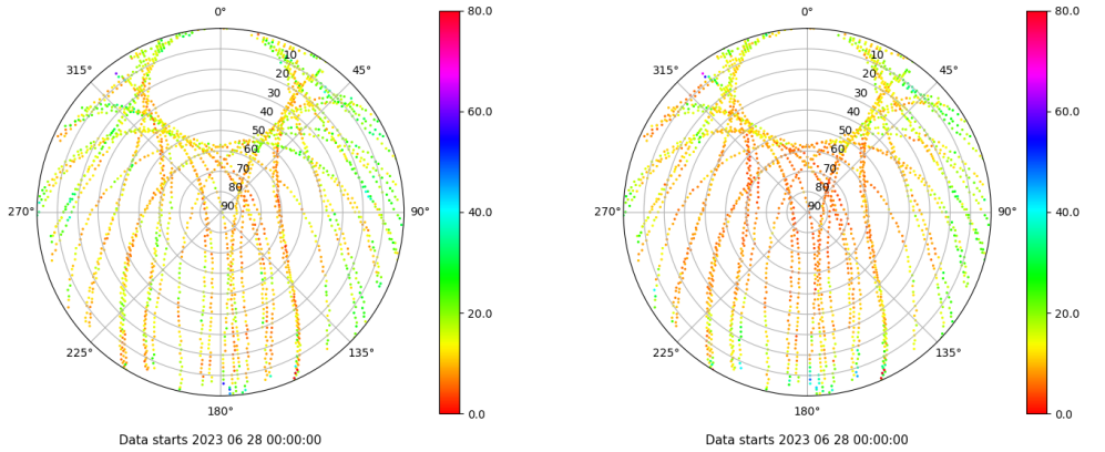
Skyplot for station ALOR. Parameter M1C Data file ALOR00ESP_R_2023179.xtr Skyplot for station ALOR. Parameter M2P Data file ALOR00ESP_R_2023179.xtr
