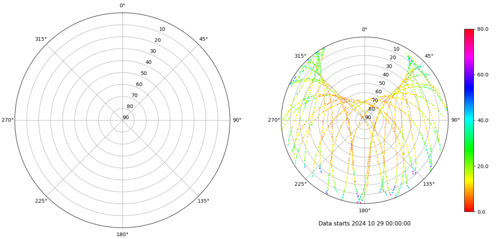
Skyplot for station ALBA. Parameter M1C Data file ALBA00ESP_R_2024303.xtr Skyplot for station ALBA. Parameter M2S Data file ALBA00ESP_R_2024303.xtr
