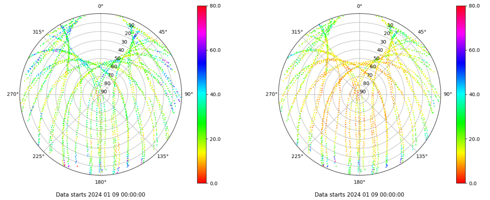
Skyplot for station ALBA. Parameter M1C Data file ALBA00ESP_R_2024009.xtr Skyplot for station ALBA. Parameter M2C Data file ALBA00ESP_R_2024009.xtr
