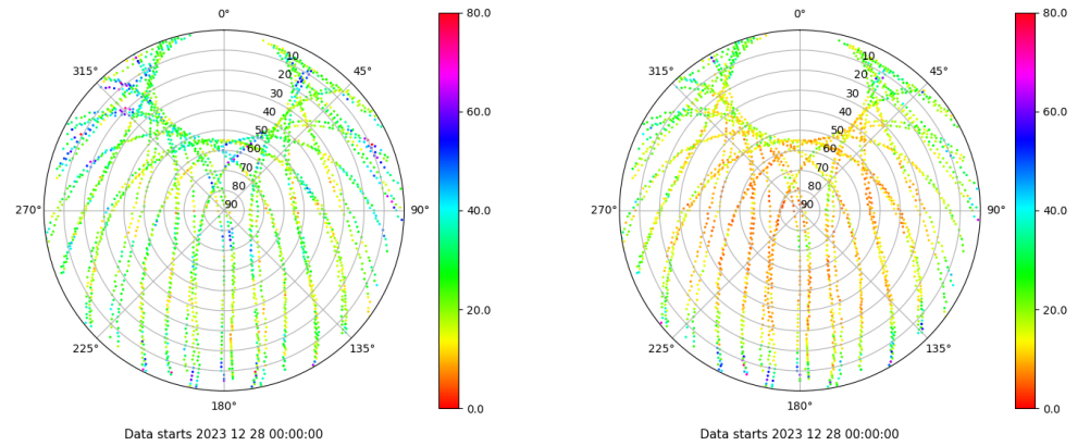
Skyplot for station ALBA. Parameter M1C Data file ALBA00ESP_R_2023362.xtr Skyplot for station ALBA. Parameter M2C Data file ALBA00ESP_R_2023362.xtr
