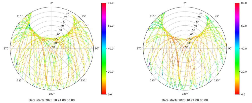
Skyplot for station ALBA. Parameter M1C Data file ALBA00ESP_R_2023297.xtr Skyplot for station ALBA. Parameter M2S Data file ALBA00ESP_R_2023297.xtr
