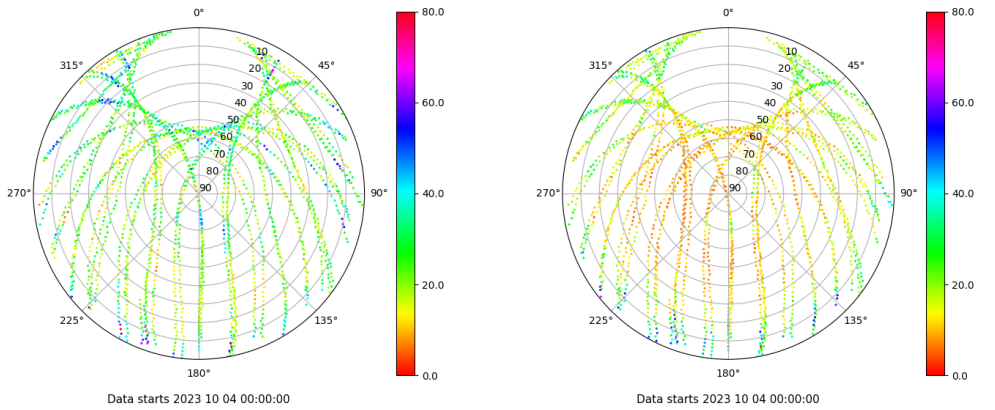
Skyplot for station ALBA. Parameter M1C Data file ALBA00ESP_R_2023277.xtr Skyplot for station ALBA. Parameter M2C Data file ALBA00ESP_R_2023277.xtr
