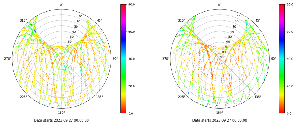
Skyplot for station ALBA. Parameter M1C Data file ALBA00ESP_R_2023270.xtr Skyplot for station ALBA. Parameter M2S Data file ALBA00ESP_R_2023270.xtr
