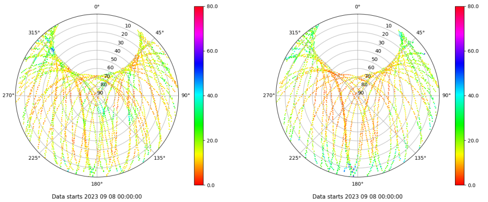
Skyplot for station ALBA. Parameter M1C Data file ALBA00ESP_R_2023251.xtr Skyplot for station ALBA. Parameter M2S Data file ALBA00ESP_R_2023251.xtr
