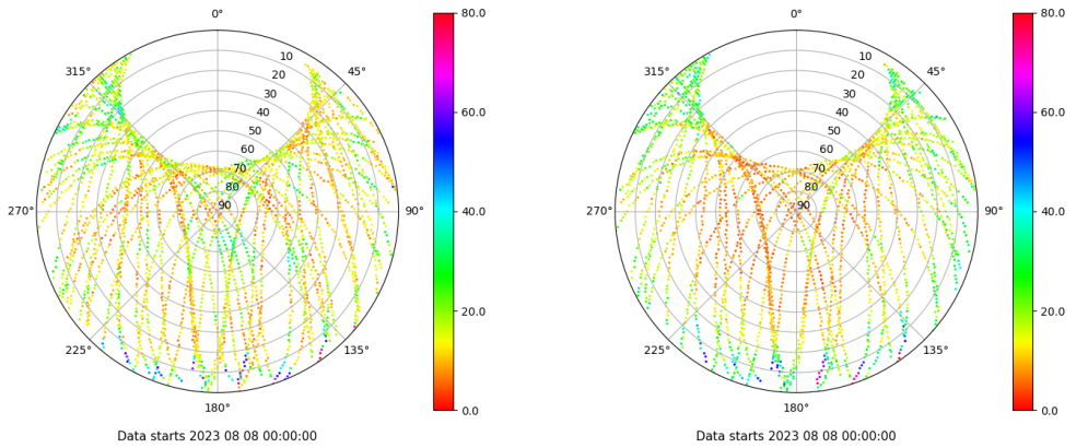
Skyplot for station ALBA. Parameter M1C Data file ALBA00ESP_R_2023220.xtr Skyplot for station ALBA. Parameter M2S Data file ALBA00ESP_R_2023220.xtr
