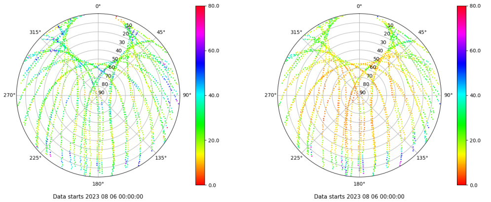
Skyplot for station ALBA. Parameter M1C Data file ALBA00ESP_R_2023218.xtr Skyplot for station ALBA. Parameter M2C Data file ALBA00ESP_R_2023218.xtr
