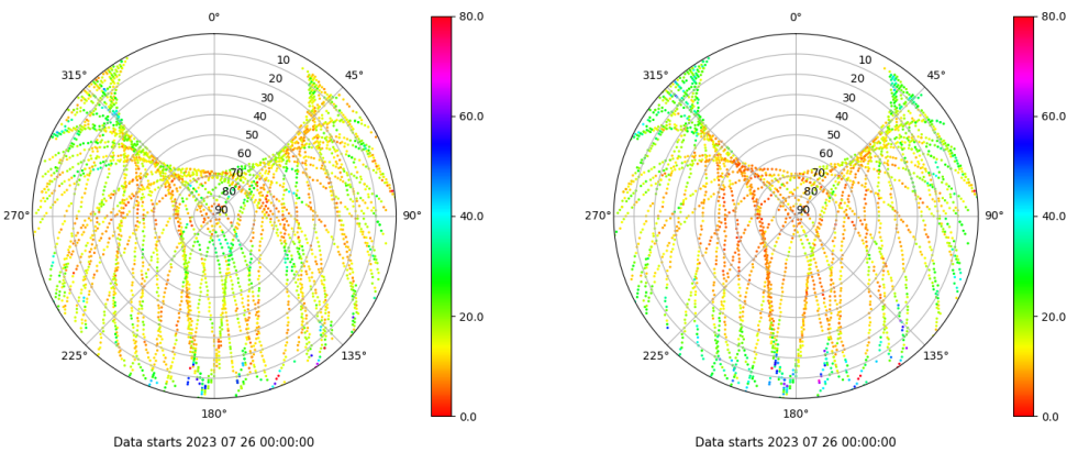
Skyplot for station ALBA. Parameter M1C Data file ALBA00ESP_R_2023207.xtr Skyplot for station ALBA. Parameter M2S Data file ALBA00ESP_R_2023207.xtr
