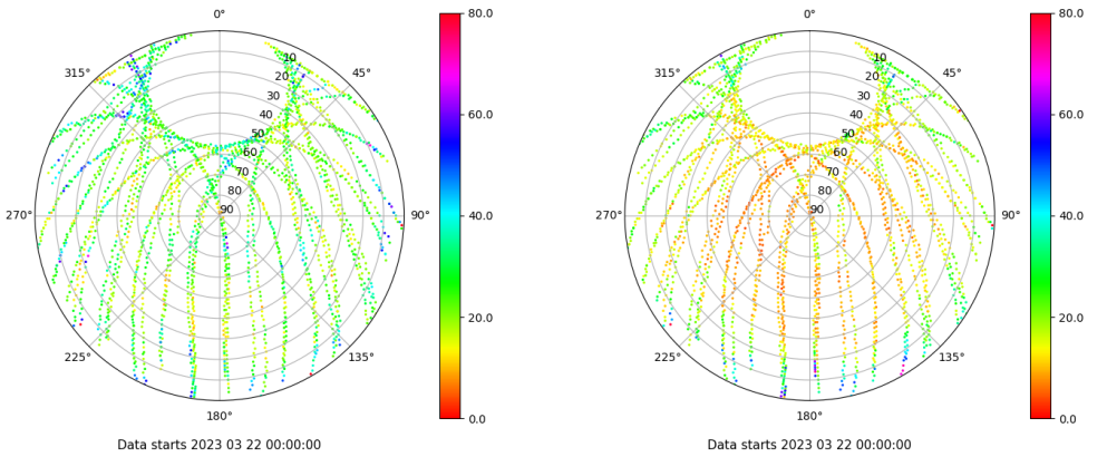
Skyplot for station ALBA. Parameter M1C Data file ALBA00ESP_R_2023081.xtr Skyplot for station ALBA. Parameter M2C Data file ALBA00ESP_R_2023081.xtr
