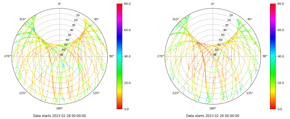
Skyplot for station ALBA. Parameter M1C Data file ALBA00ESP_R_2023059.xtr Skyplot for station ALBA. Parameter M2S Data file ALBA00ESP_R_2023059.xtr
