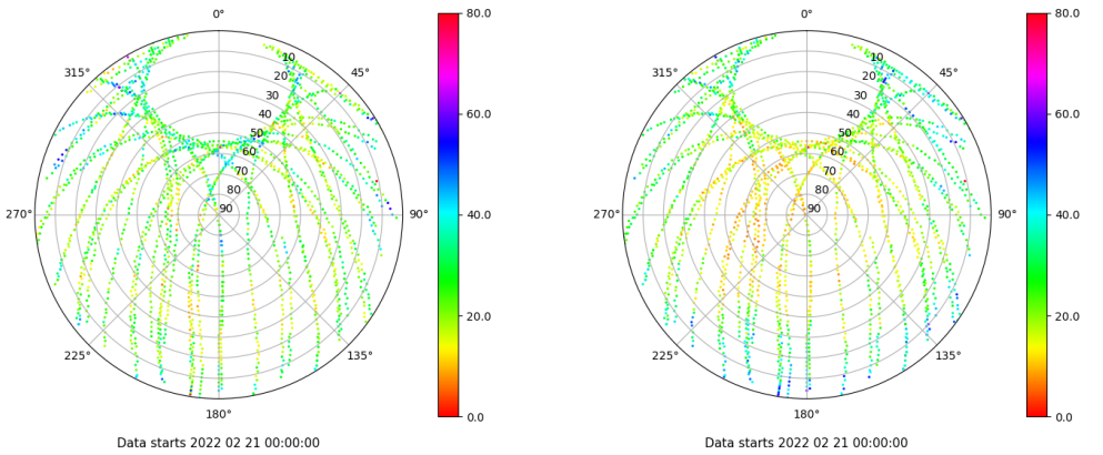
Skyplot for station ALBA. Parameter M1C Data file ALBA00ESP_R_2022052.xtr Skyplot for station ALBA. Parameter M2P Data file ALBA00ESP_R_2022052.xtr
