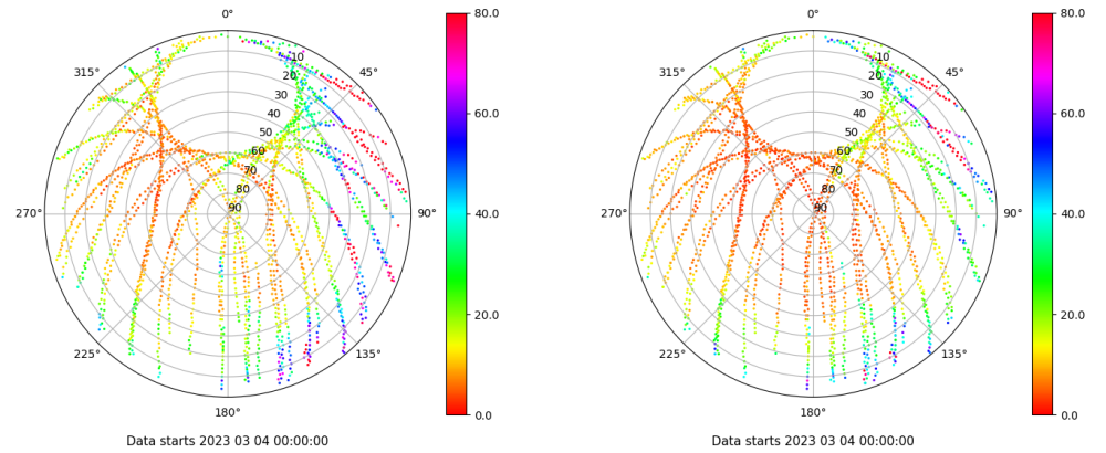
Skyplot for station ACOR. Parameter M1C Data file ACOR00ESP_R_2023063.xtr Skyplot for station ACOR. Parameter M2C Data file ACOR00ESP_R_2023063.xtr
