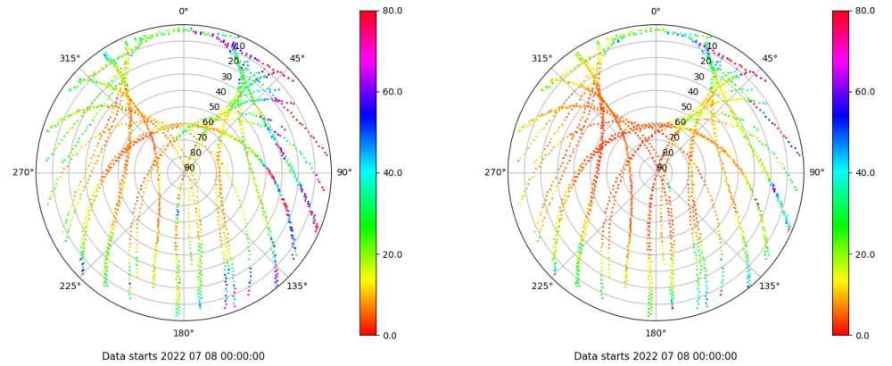
Skyplot for station ACOR. Parameter M1C Data file ACOR00ESP_R_2022189.xtr Skyplot for station ACOR. Parameter M2C Data file ACOR00ESP_R_2022189.xtr
